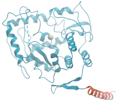
human PAH (2pah)
