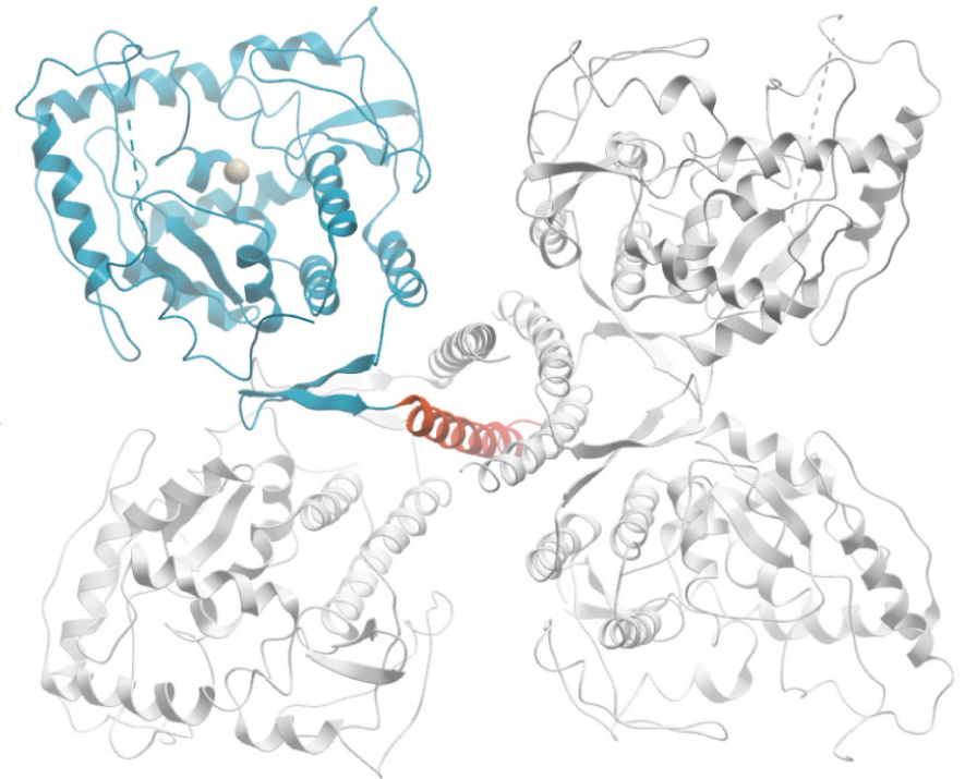
human PAH (2pah) tetramer
